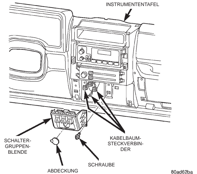
Abb. 6 Schaltergruppenblende
